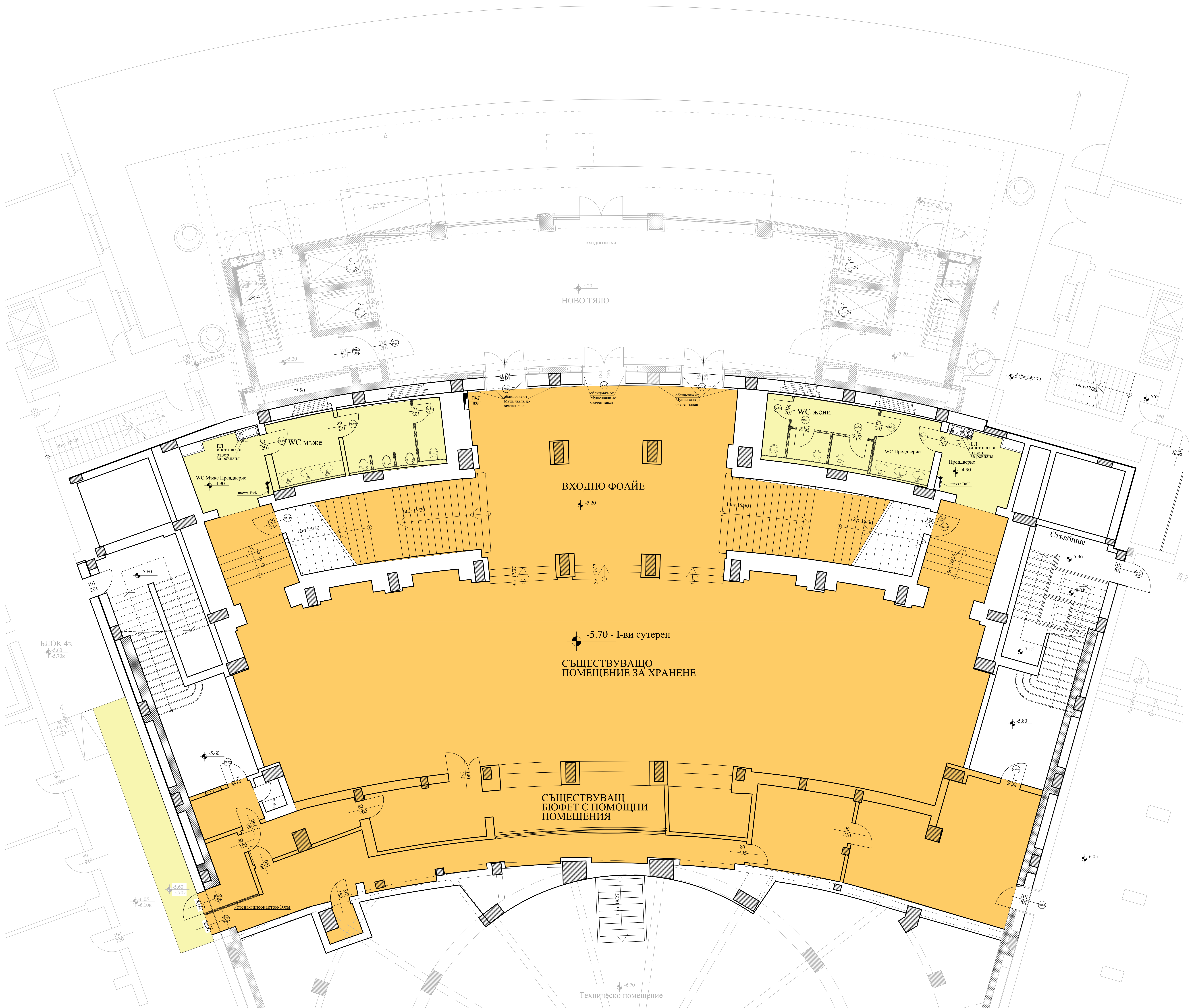
СЪЩЕСТВУВАЩО ПОЛОЖЕНИЕ АРХИТЕКТУРНО РАЗПРЕДЕЛЕНИЕ НА ЧАСТ ОТ I-ВИ СУТЕРЕН -5.70, КЪДЕТО Е РАЗПОЛОЖЕН БЮФЕТЪТ С ПОМЕЩЕНИЕТО ЗА ХРАНЕНЕ
