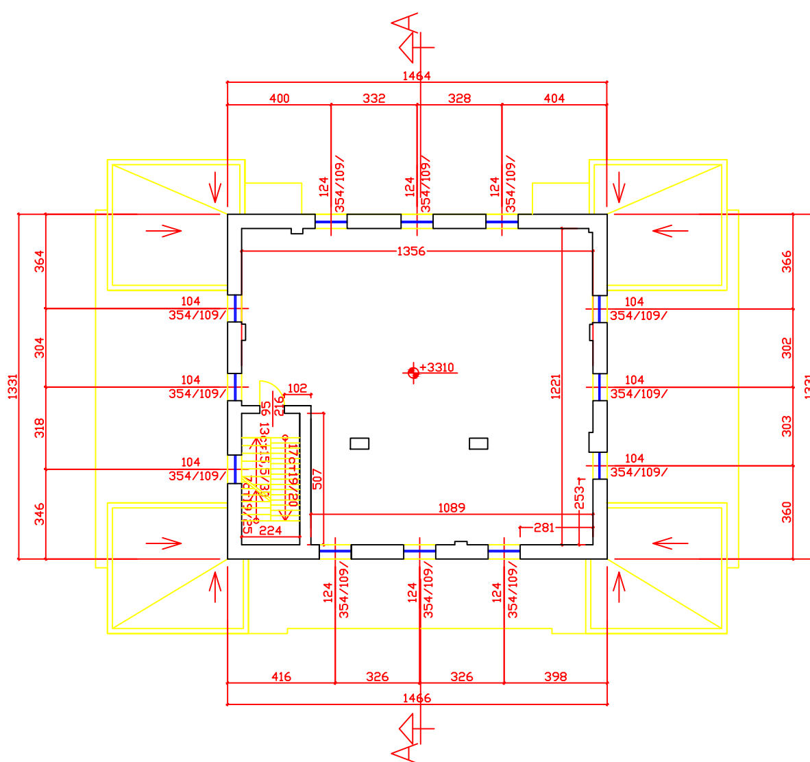
СЕДМИ ЕТАЖ М 1:200
