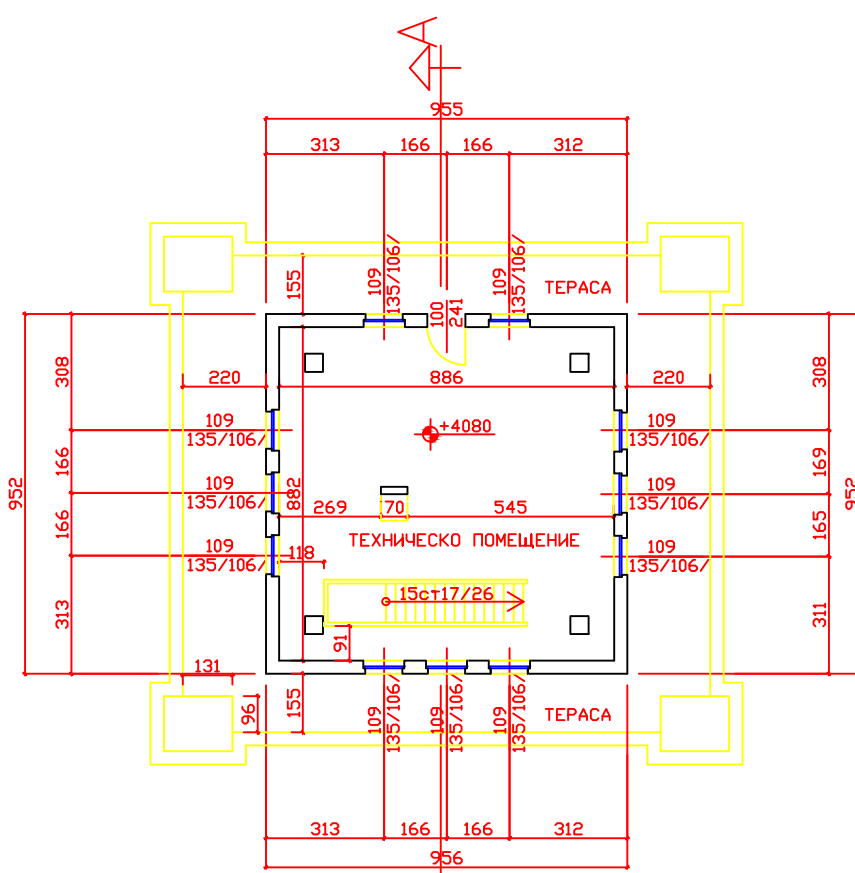
ДЕВЕТИ ЕТАЖ М 1:200
