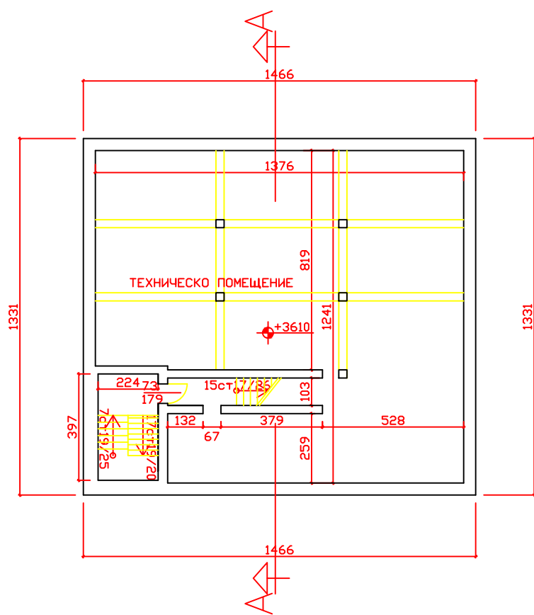
ОСМИ ЕТАЖ М 1:200
