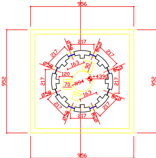
ДЕСЕТИ ЕТАЖ М 1:200
